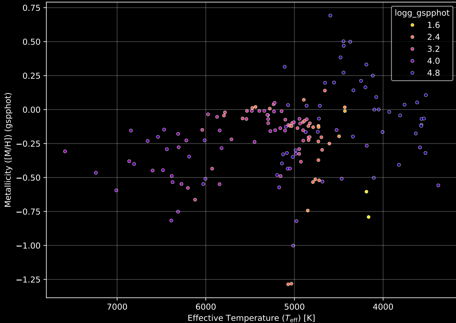
APOGEE DR17 Field: [120-45] Stellar Population Parameters (n= 159)
